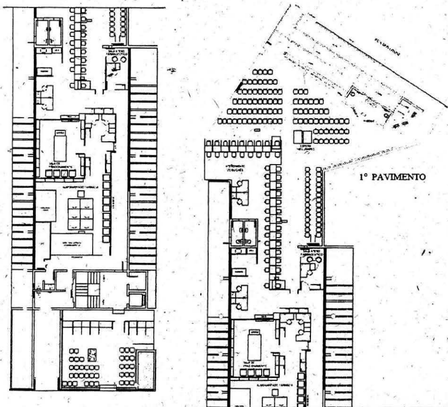
Figura 1 – Layouts do 1º pavimento (Lado Av. Brasil e lado R. dos Otoni)
