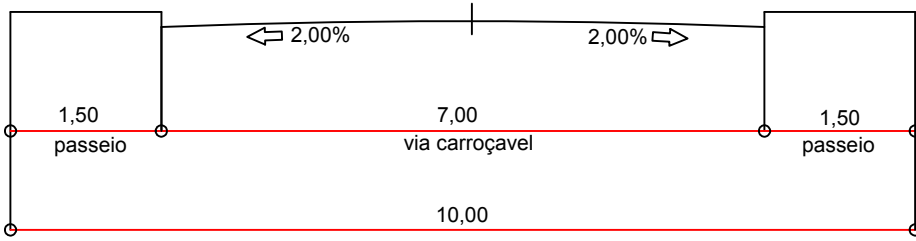
PERFIL TRANSVERSAL DO ARRUAMENTO
